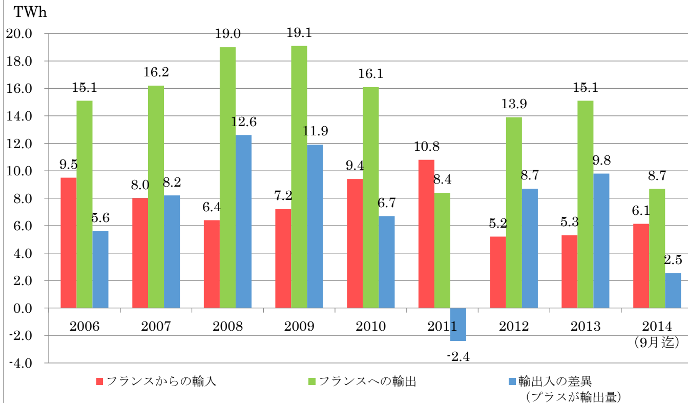
図1：ドイツの電力輸出入量（対フランス）
